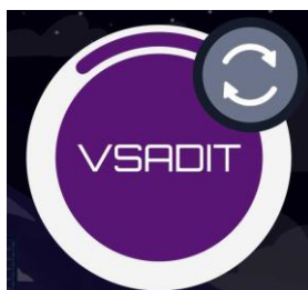
Obrázek 1: tlačítko VSADIT
