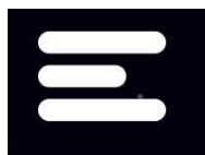
Obrázek 6: tlačítko MENU
